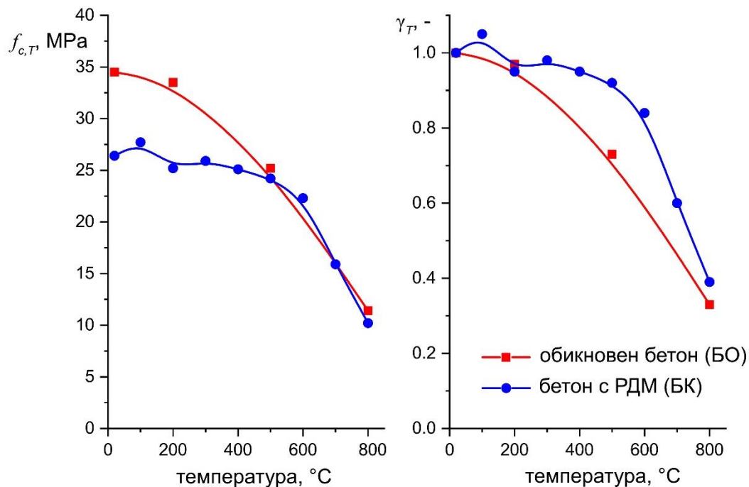
Фигура 1. Изменение на якостта на натиск f_{c,T} и коефициента на редукция на якостта на натиск, \gamma_T , на бетон с естествен ЕДМ (БО) и бетон с РЕДМ (БК) при повишаване на температури
